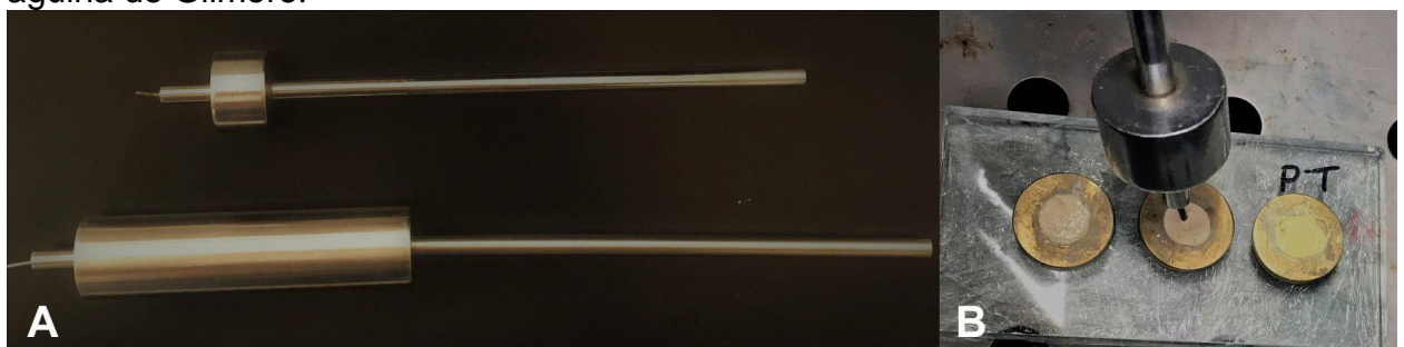
Figura 1. (A) Agulhas de Gilmore de 113,5g para determinar a presa inicial e a de 453,5g para a presa final dos espécimes. (B) Mensuração do tempo de presa com a agulha de Gilmore.
